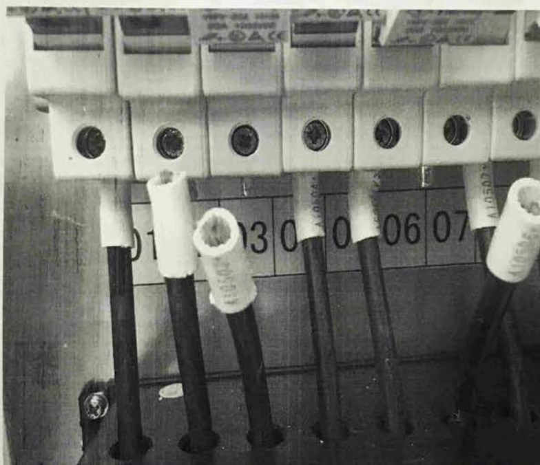
接线端子连接不合格轻松拽出
