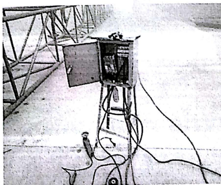
配电箱无接地、接线不规范
