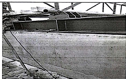
桁架梁安装严重倾斜
