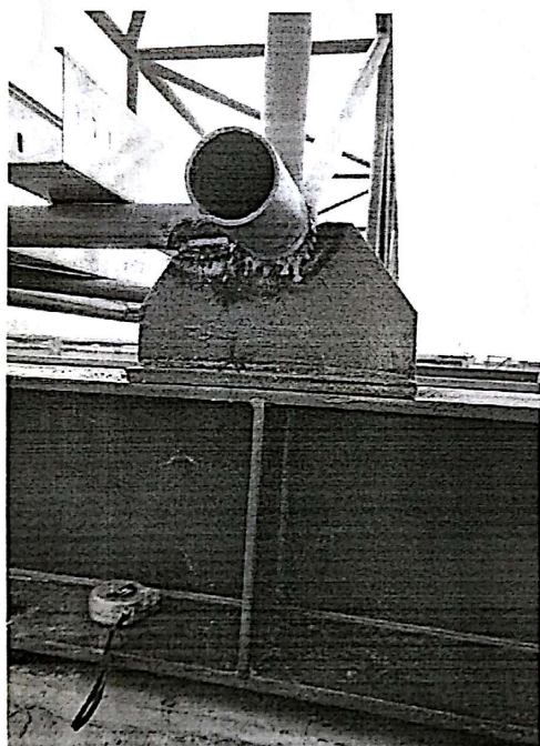
桁架与支座连接不符合图纸设计及规范要求
