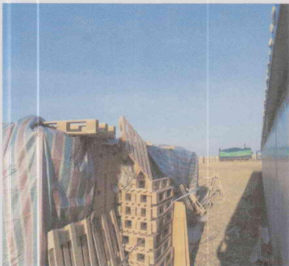
临舍区材料已进行清理、并使用安全警示带进行维护
