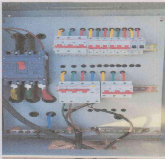
按照“一机 一闸 一漏 一箱”配备电箱
