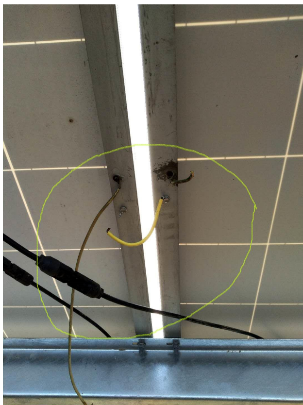
组件间接地已断开
