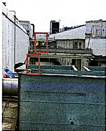
植筋位置偏离
