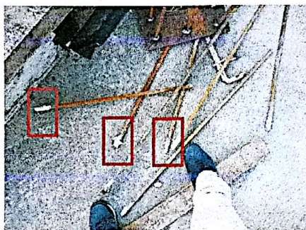
植筋深度太浅
