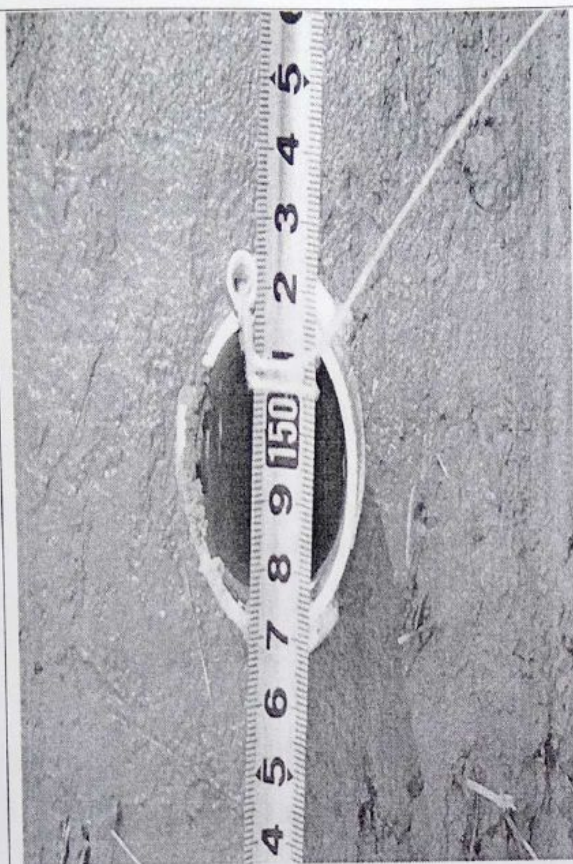
地锚桩间距（整改后）03.22
