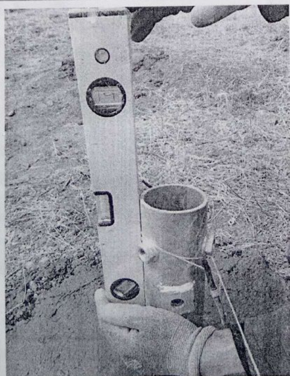
地锚桩垂直度测量 03.22
