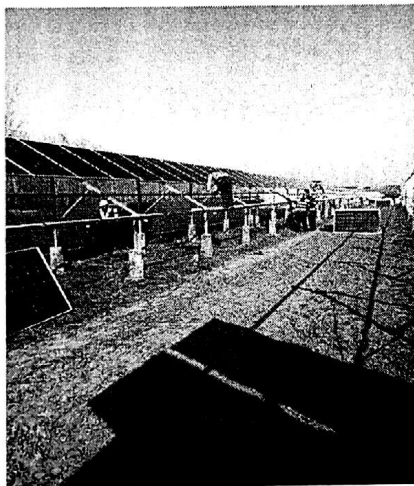
施工人员踩踏檩条
