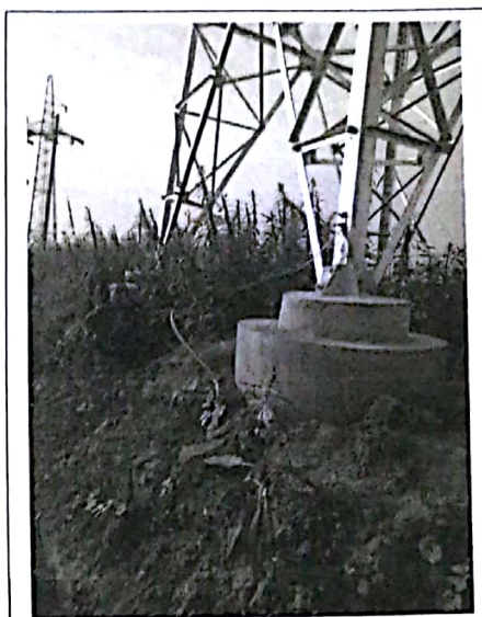
外线接地不符合规范
