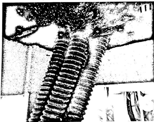
12、 箱逆变接地网焊接处防腐不到位。
