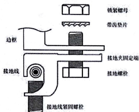
图 7 安装方式
