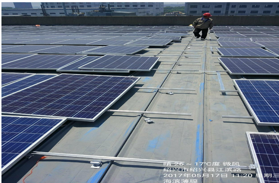
组件放置方式不当划伤背板
