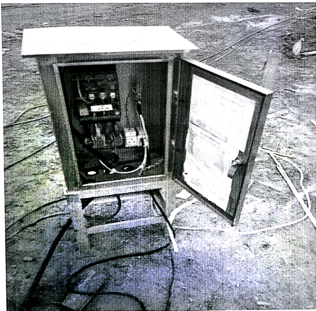
配电箱进行更换并做好箱体接地
