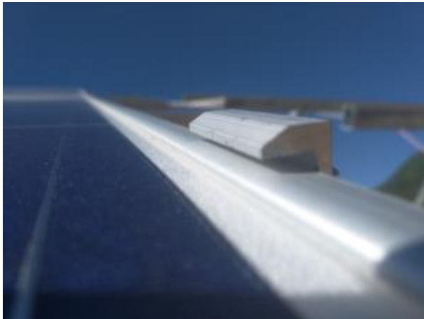
边压块安装不符合要求（未压靠、歪斜）
