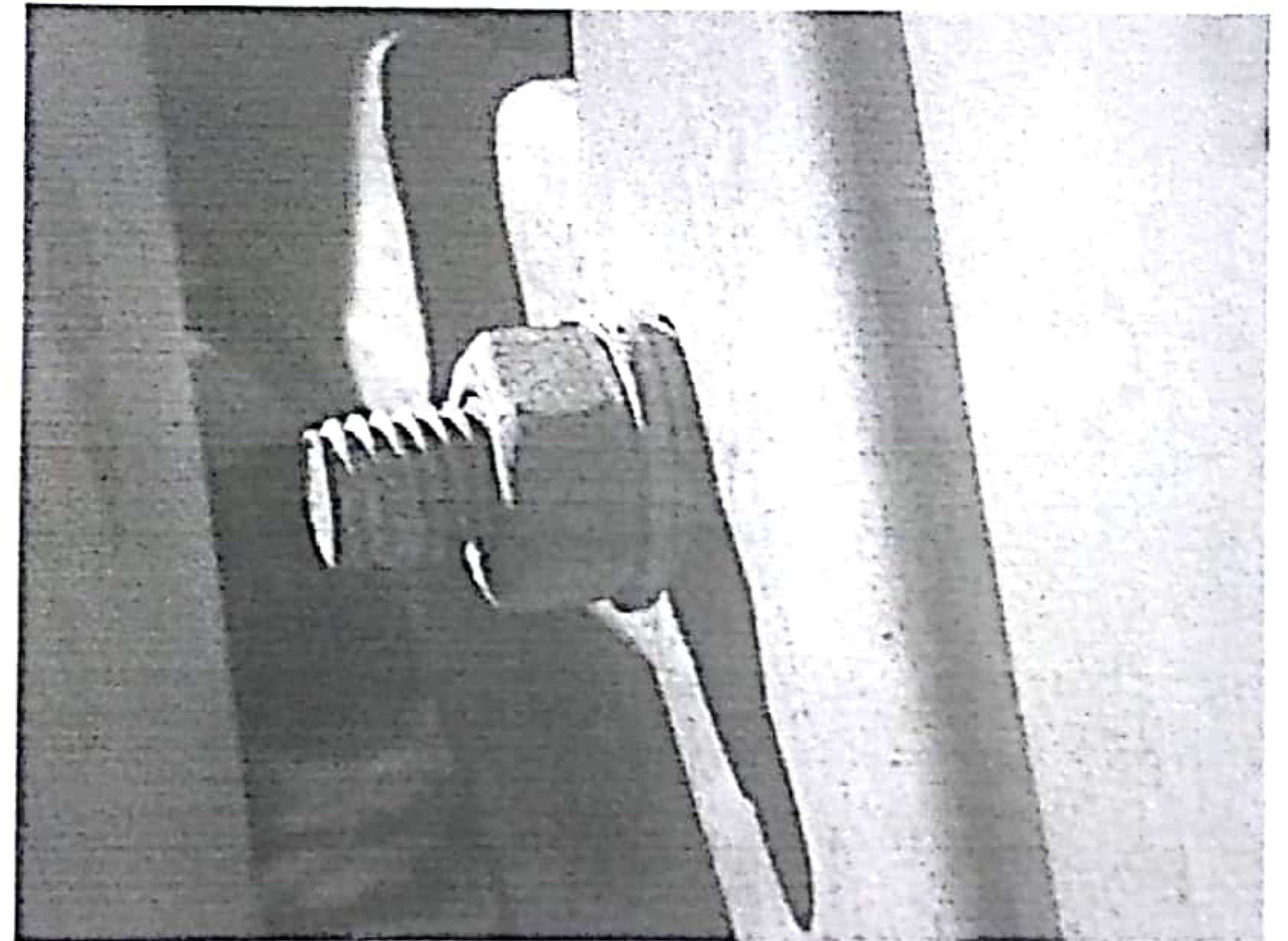
螺栓的垫片与弹垫位置错误或无垫片、弹垫
