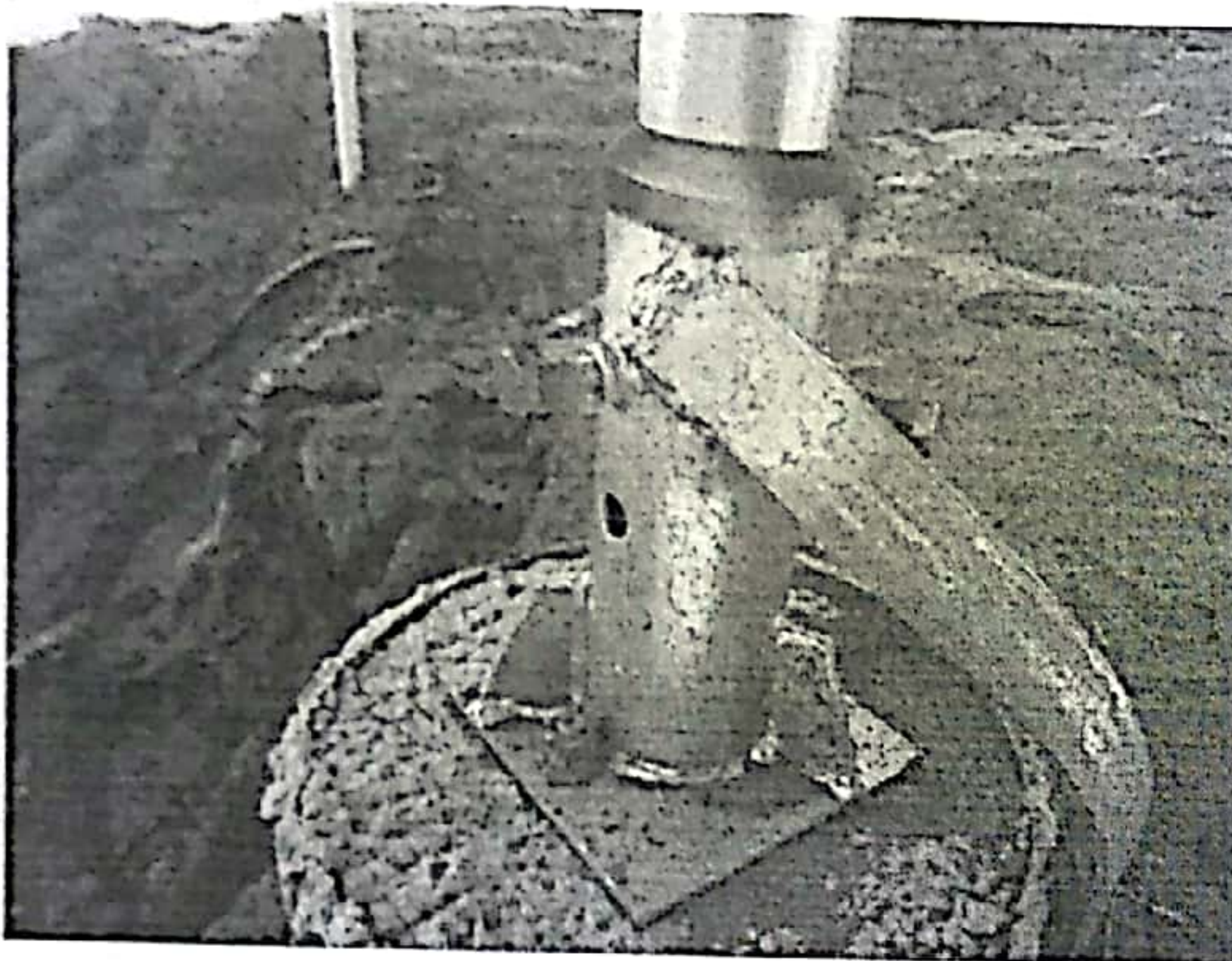
接地扁铁焊接不规范、焊接区长度不足
