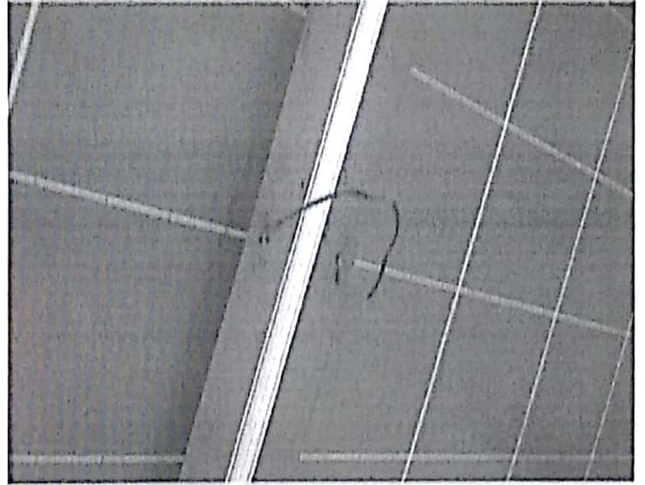
组件、组件与支架接地未连接
