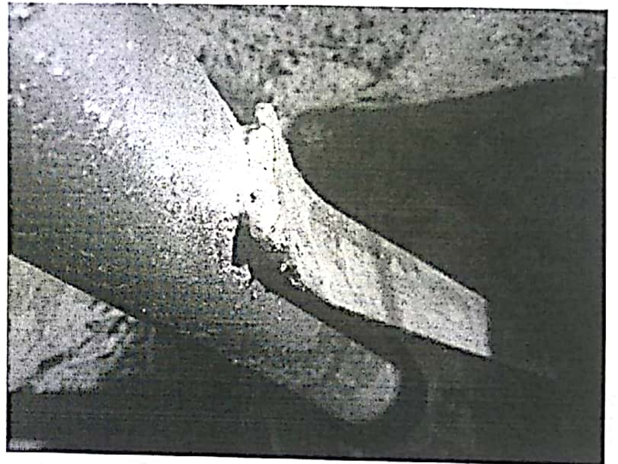
接地扁铁焊接不规范、焊接区长度不足
