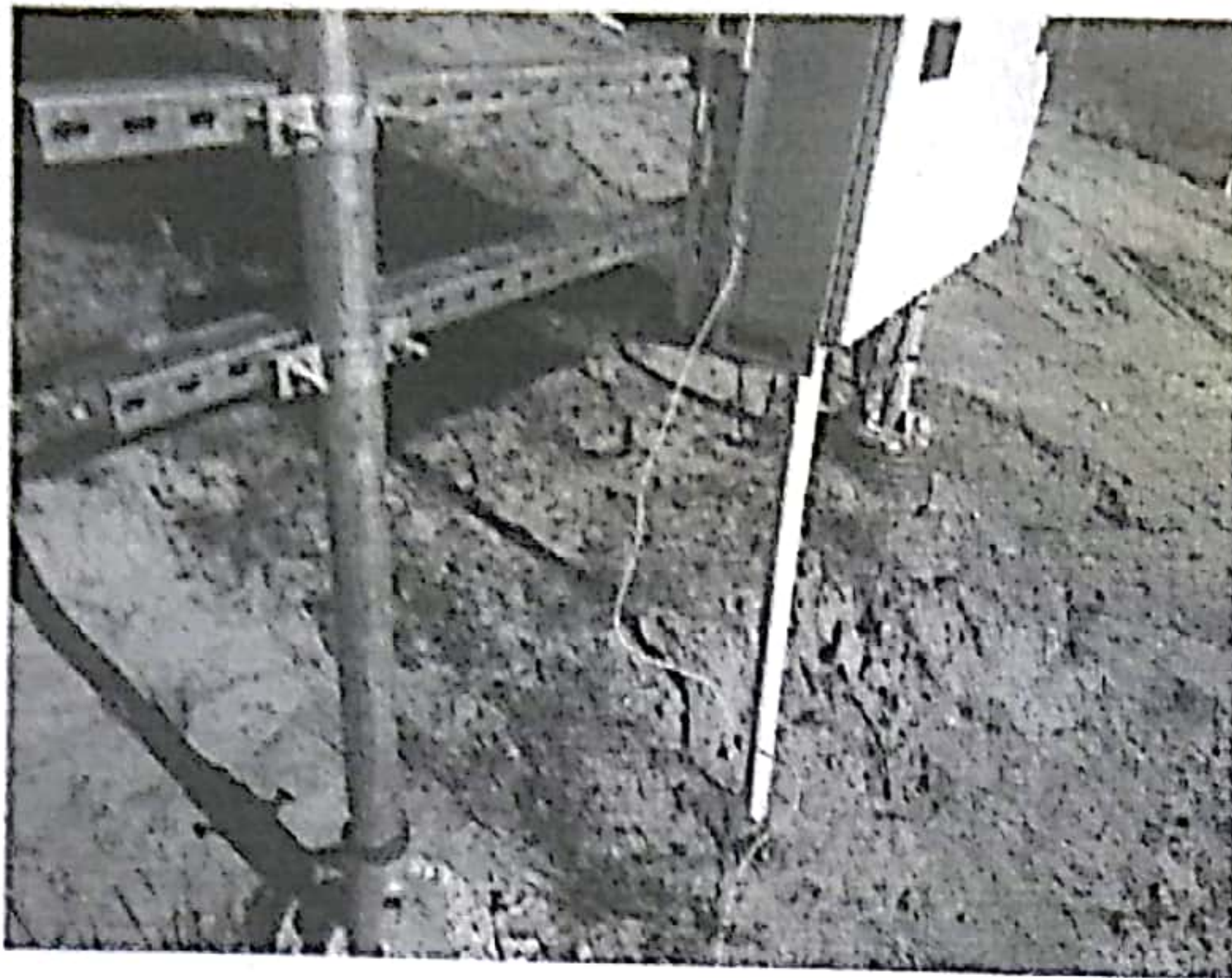
箱体接地线不规范
