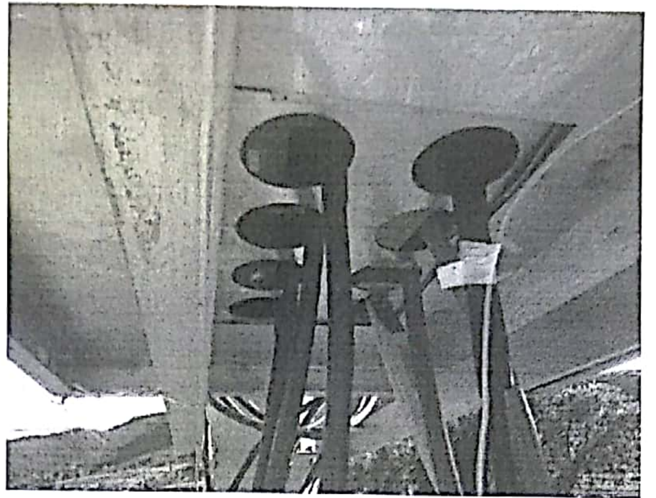
防孤岛保护箱洞口未封堵
