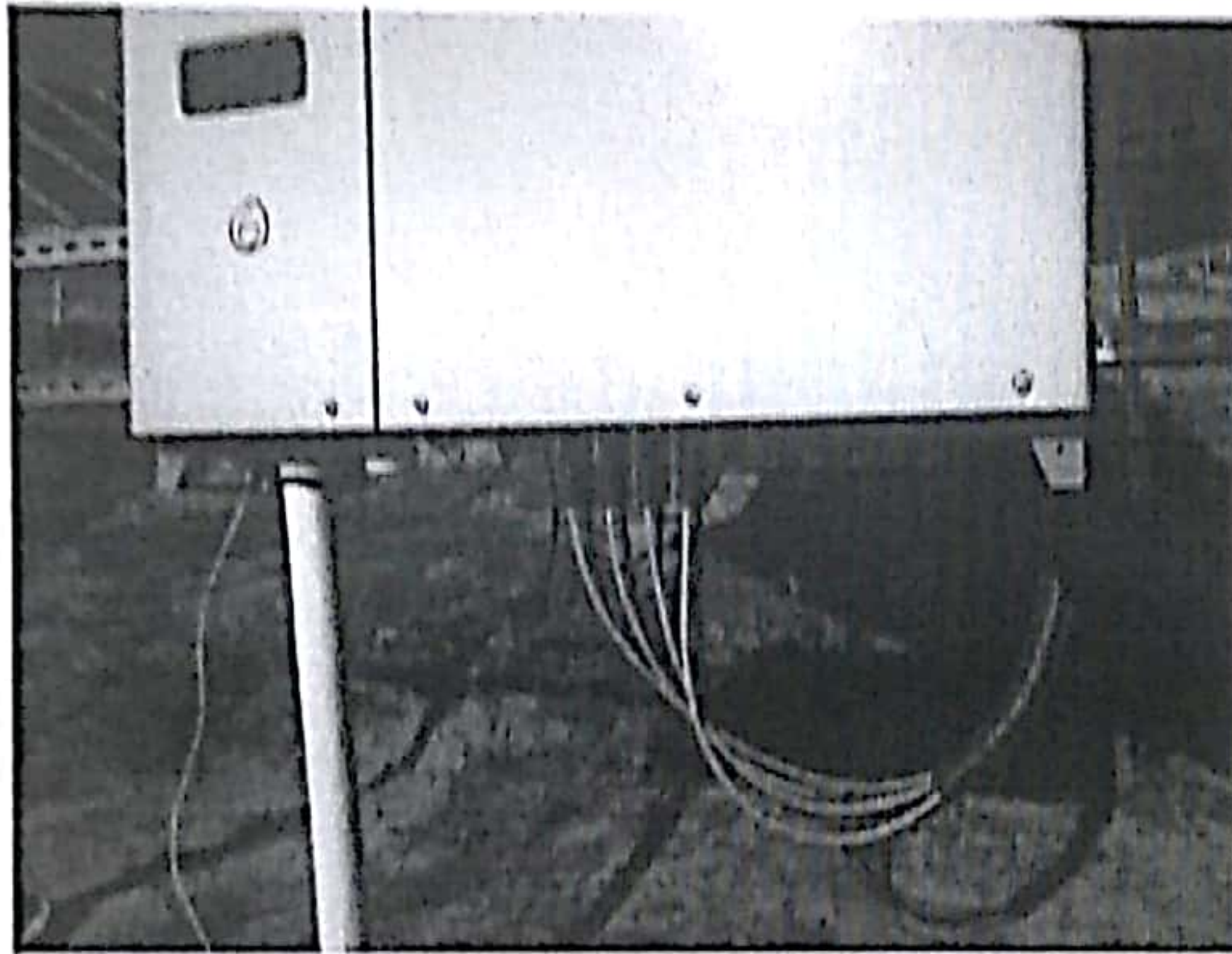
逆变箱体进线套管过短、电缆线混乱不规范
