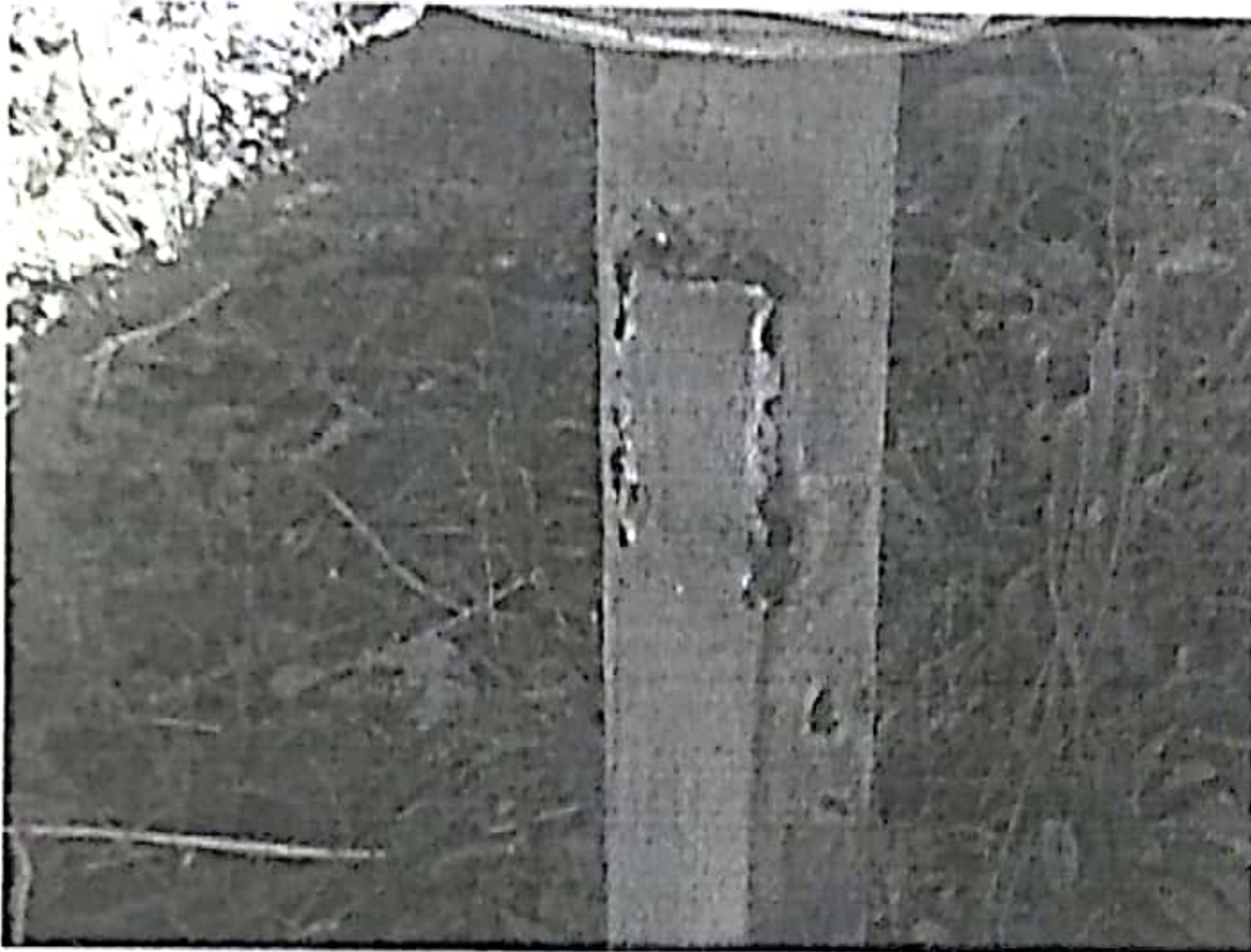
接地扁铁焊接区未刷防腐
