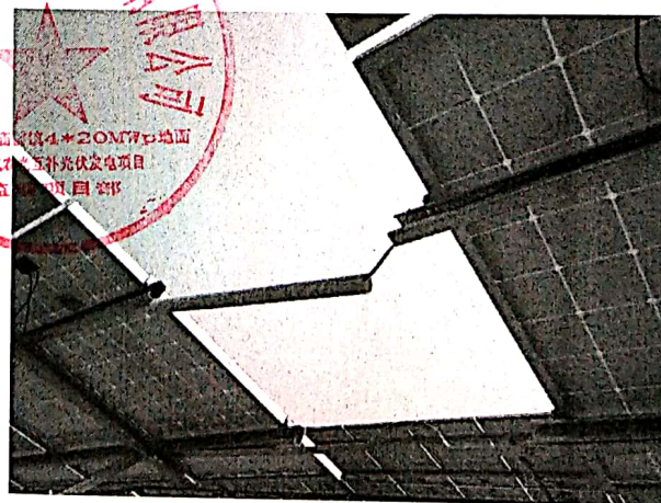
组串间光伏电缆套管未固定、防火封堵
