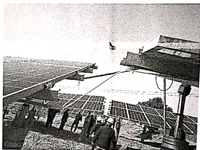
支架接地连接不符合设计图纸要求
