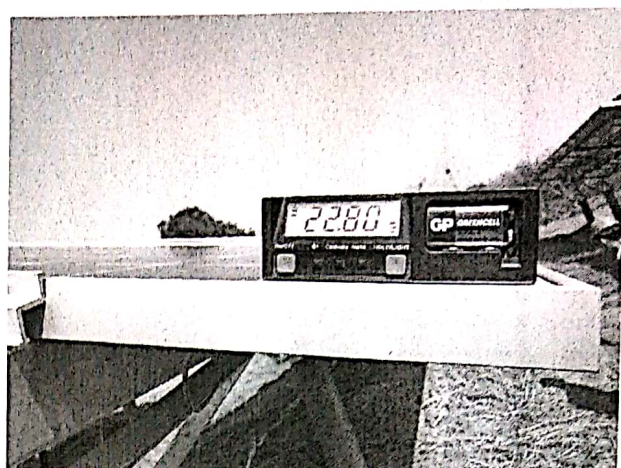
组件安装角度 22.8 度
