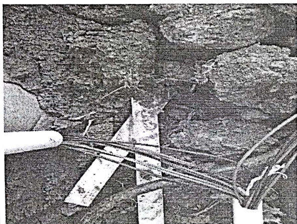
40 区接地扁铁搭接长度偏短未防腐
