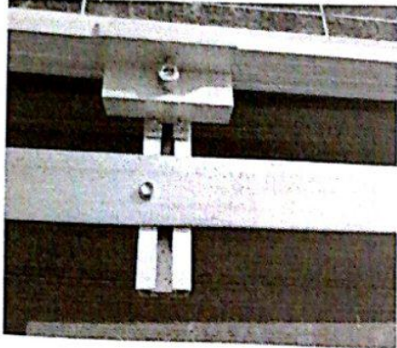
接地扁铁固定时铁屑未清理干净，产生锈迹
