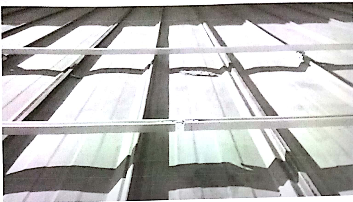
檩条连接处缝隙太大
