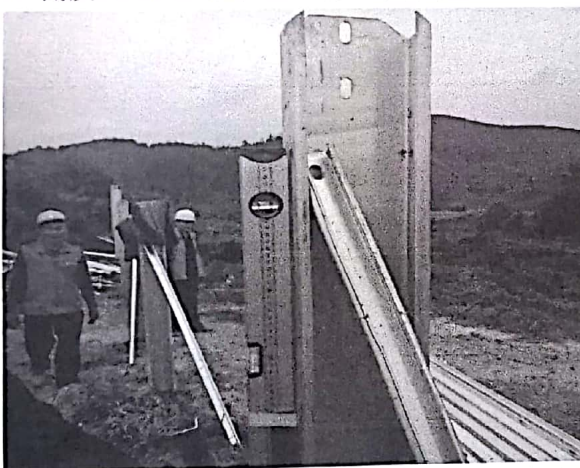
3. 立柱安装已垂直，安装距离已经整改，已达到图纸设计的要求。
