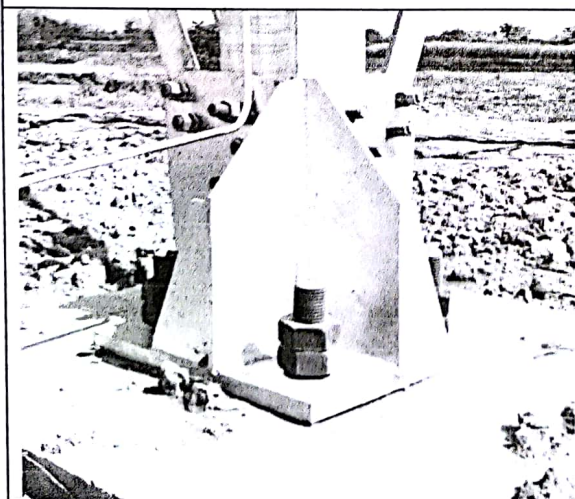
地脚螺栓螺母紧固不到位、未加平垫
