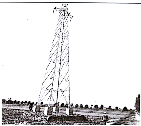
导线敷设时铁塔未采取安全保护措施
