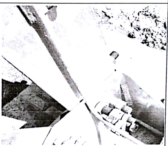
塔基底部螺母未紧固到位
