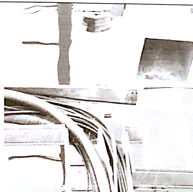
桥架转弯处里面电缆未设保护措施
