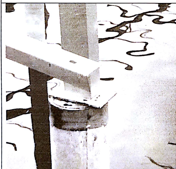
个别立柱没有满焊
