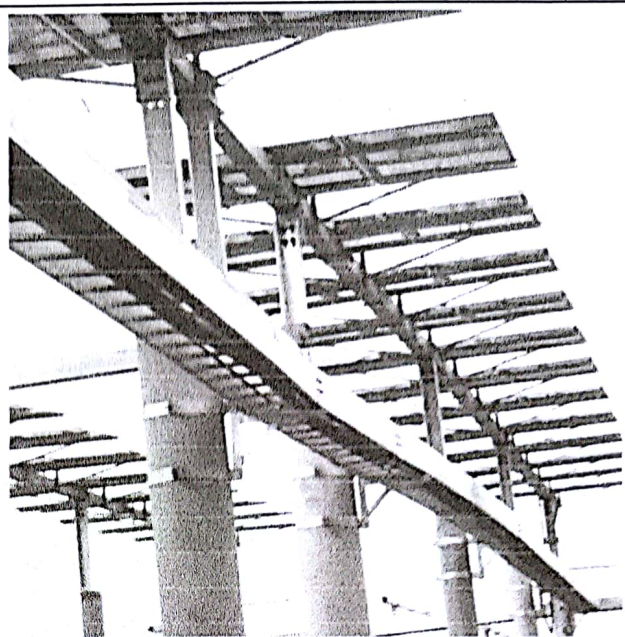
高压电缆桥架严重弯曲
