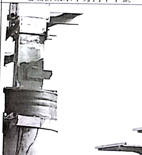
接地扁铁焊接长度不够
