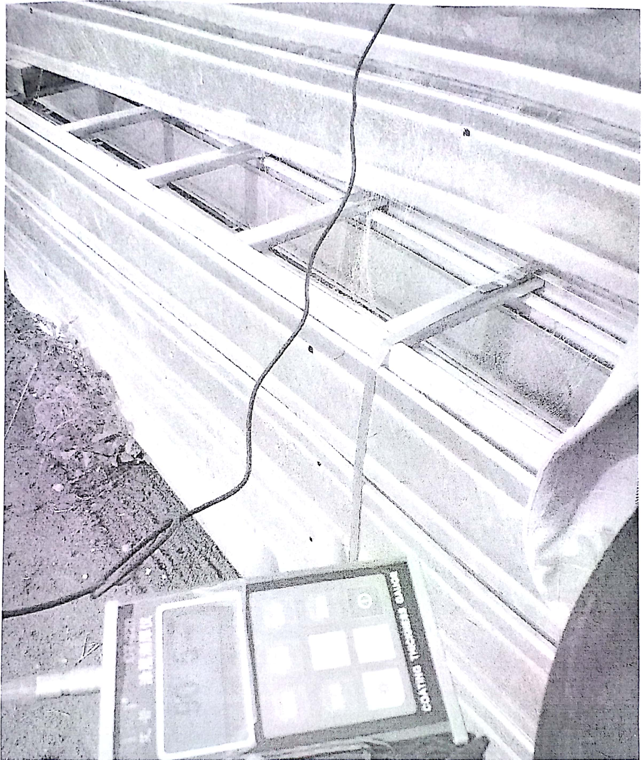
镀锌处理后桥架镀锌层检测
