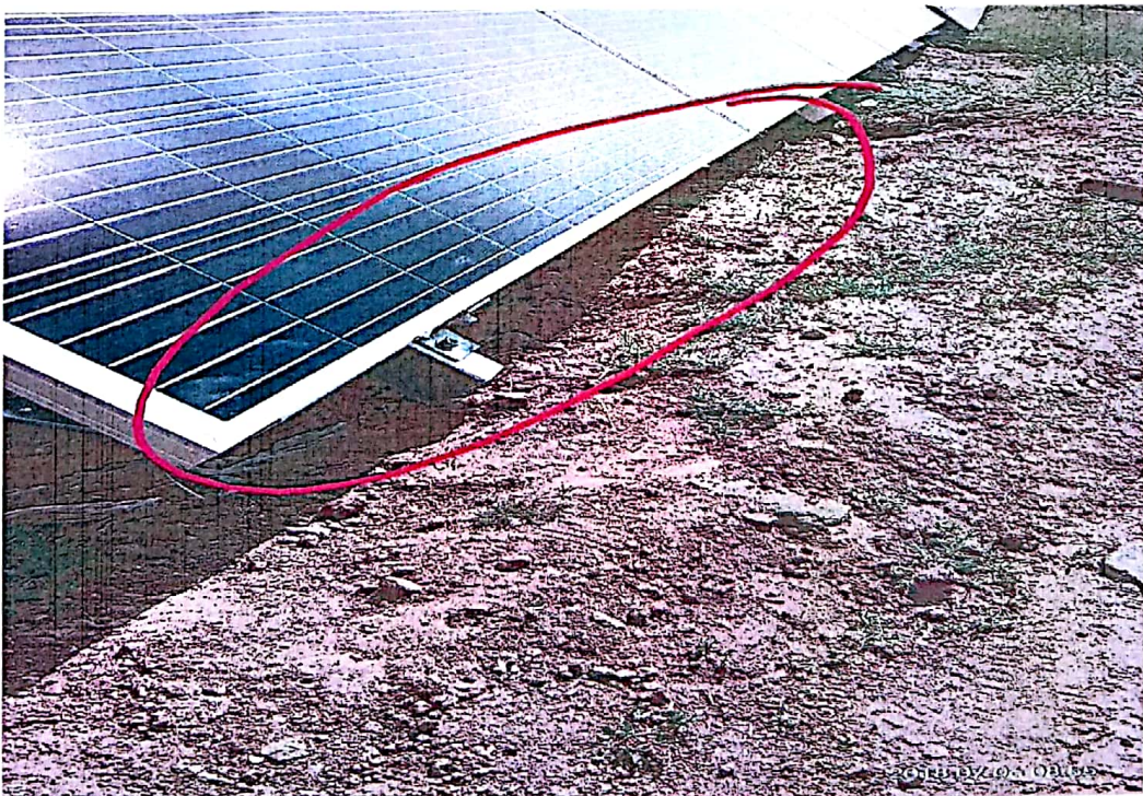
光伏支架、组件安装后
