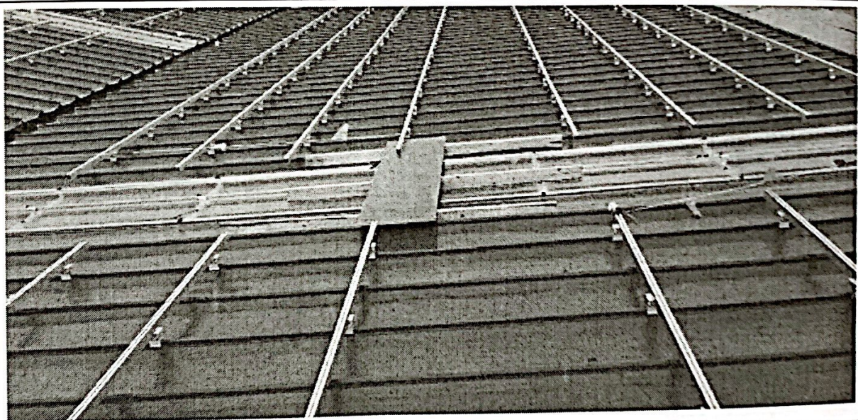
2. 施工通道处，警示带已进行分段隔离
