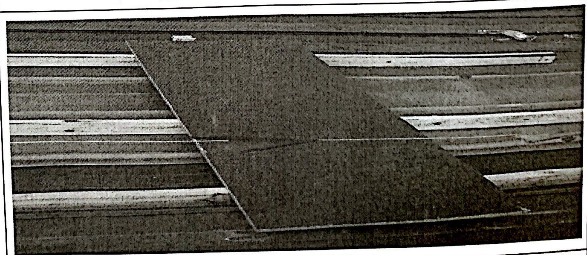
3. 屋面采光带铺设木板处已用钉子进行有效固定在木方上
