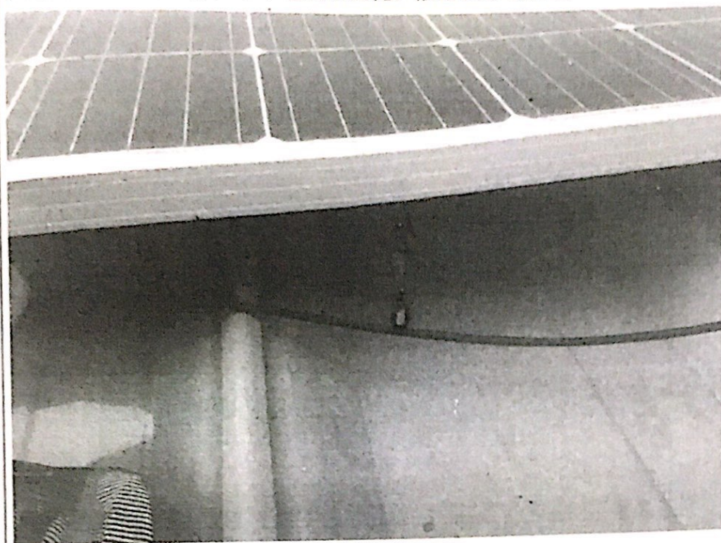
5#屋面汇流箱内有未做防火封堵现象
