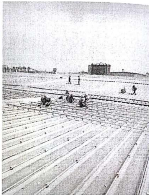
问题四：安装完成夹具、导轨的区域 采光带上安全网被拆除
