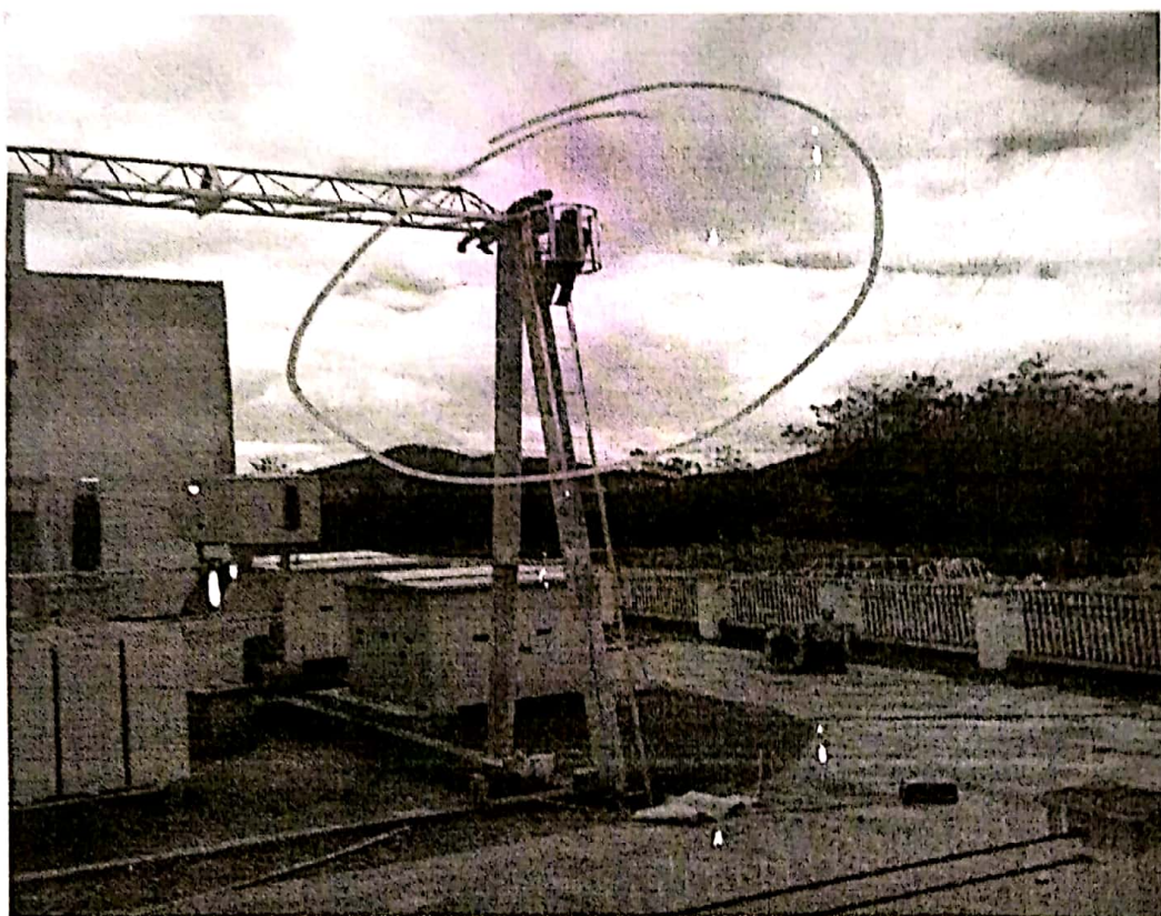
升压站内主变构架施工人员安全带配戴 (2020.4.8)
