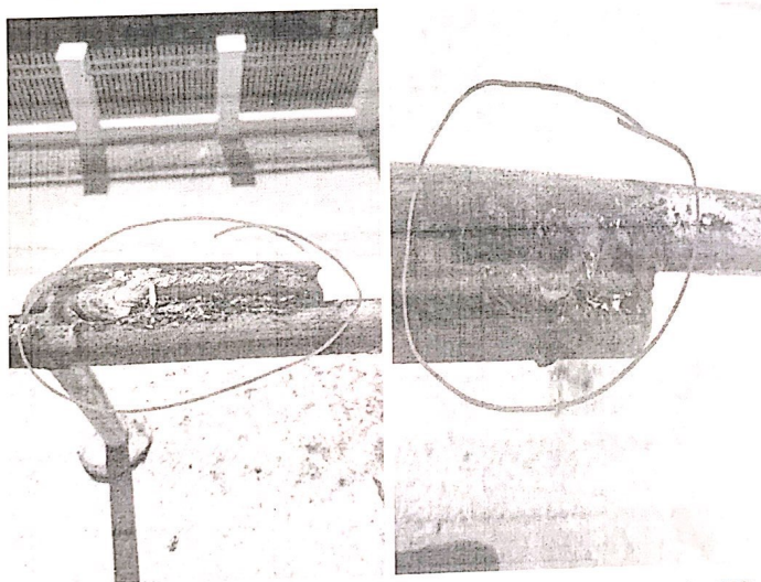
升压站综合配电楼屋顶防雷接地网（ \Phi 16 热镀锌圆钢）焊接存在漏焊、焊渣未清理现象
