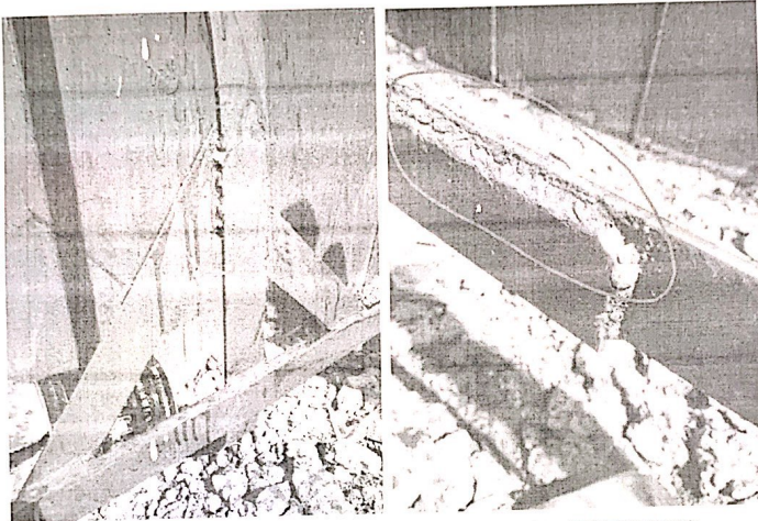
16#、17#风机基础环网接地热镀锌扁铁焊接存在漏焊、断焊、焊缝不饱满现象
