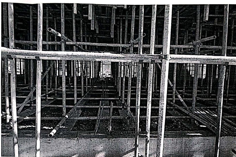
已调整 5m 范围内设置一道剪刀撑
