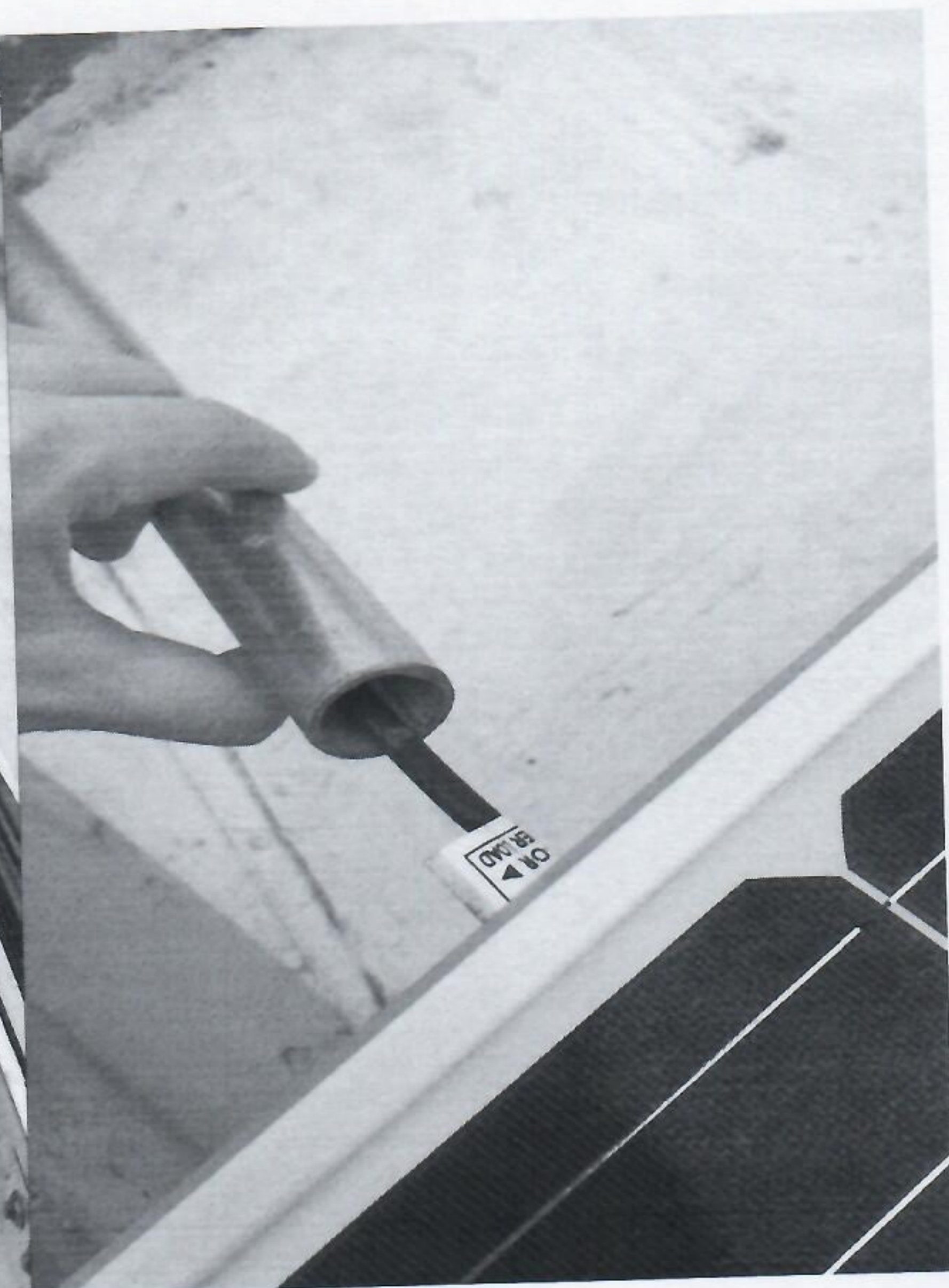
镀锌管未做钝化处理
