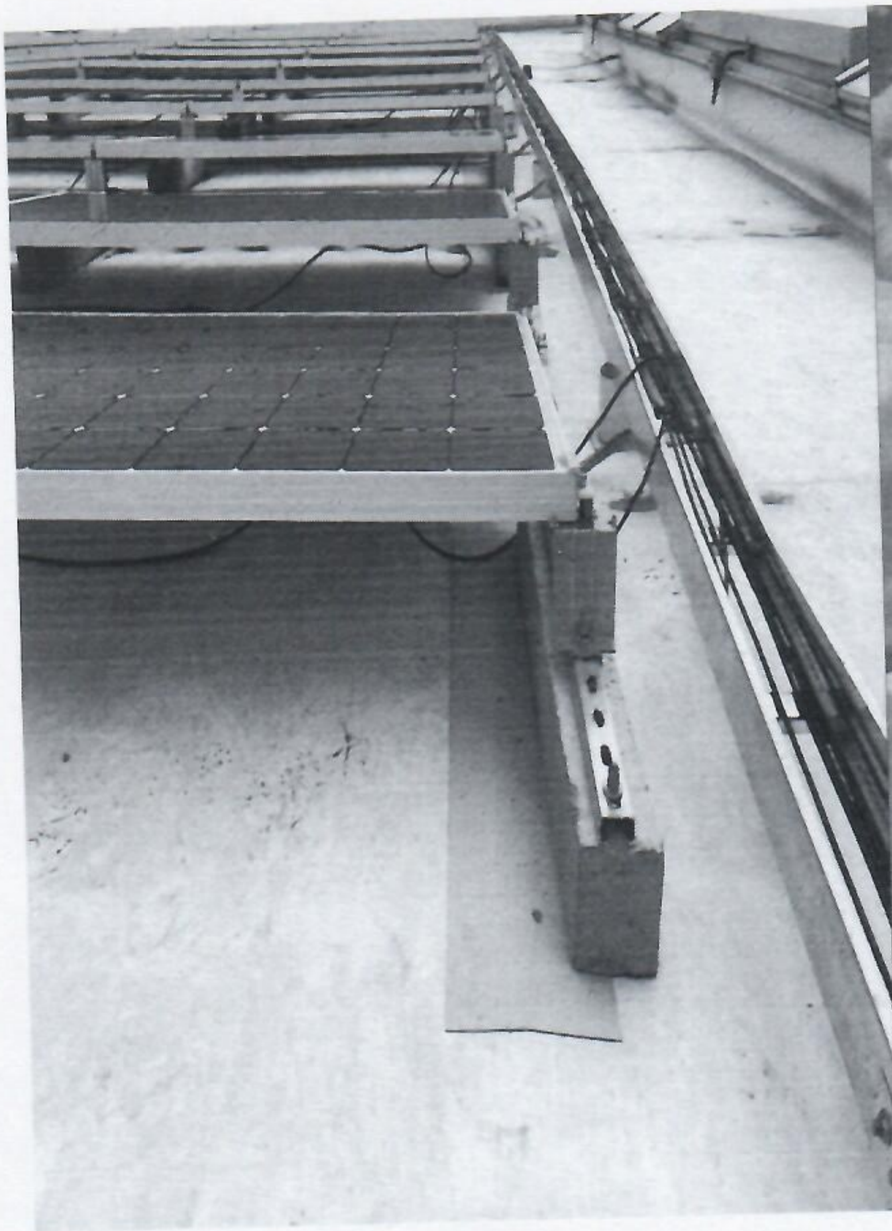
预制基础未完全摆放在 PVC 卷材上
