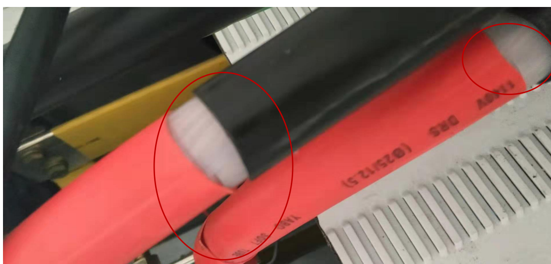
附图九：热缩管未包到位、绝缘层刀口划伤
