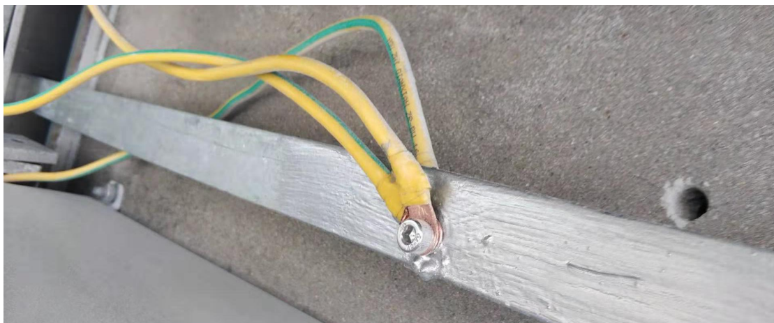
附图三：不同线径的接地线接于同一接地点
