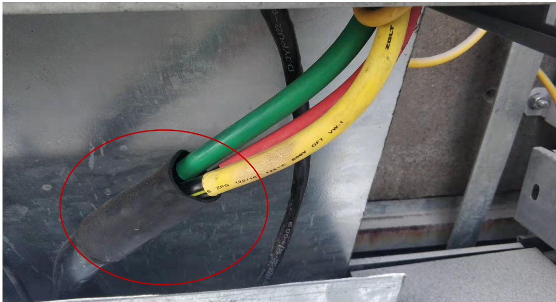
附图二：汇流箱、逆变器个别电缆头未套三只套存在隐患
