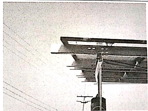
支架斜梁扭曲变形
