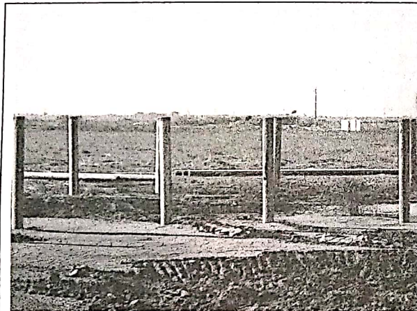
管桩桩体倾斜严重
