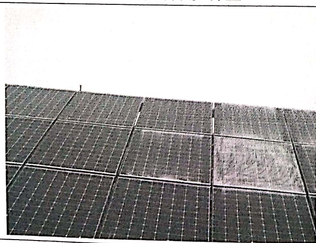
组件安装错缝严重
