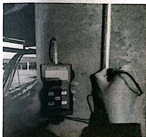
附图：圆钢镀锌层厚度不符合要求图片
