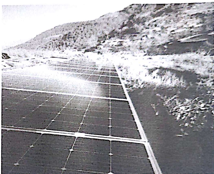
二标段支架施工
