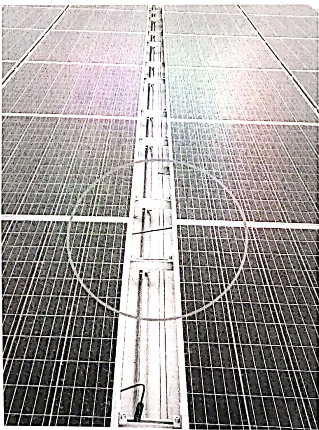
图 3: 直流电缆未穿管。
