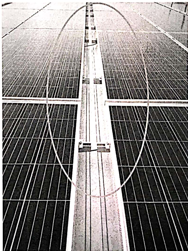
图 4: 直流电缆未穿管。
