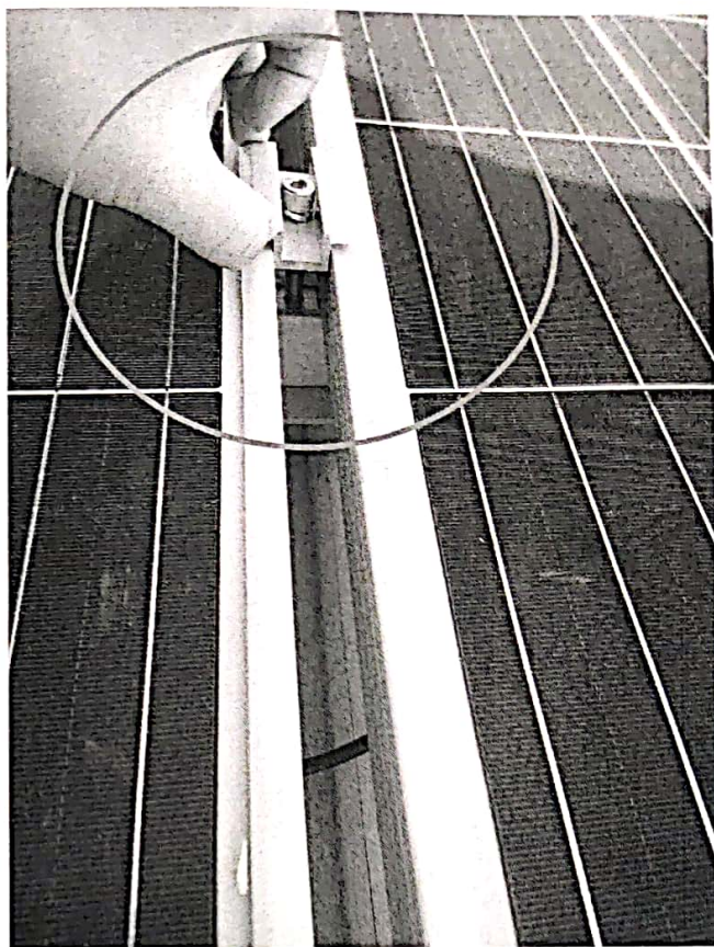
图 2: 组件压块漏压。
