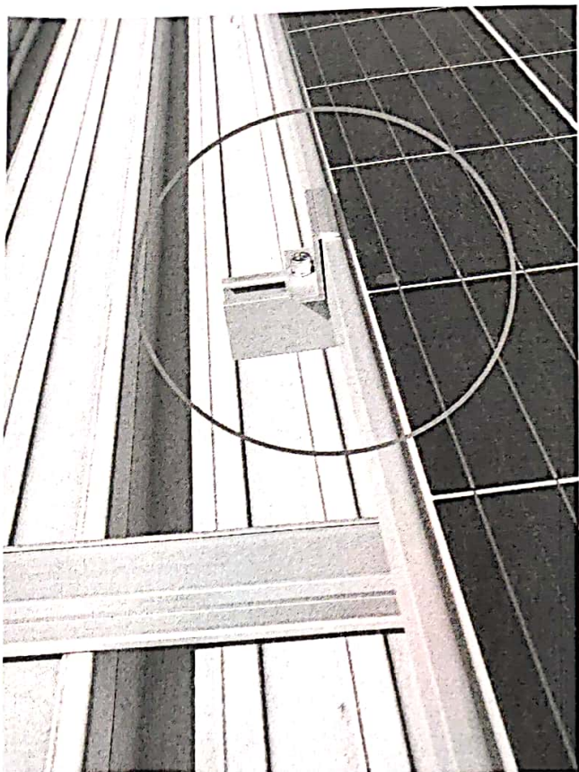
图 1: 组件压块安装不吻合不牢靠。
