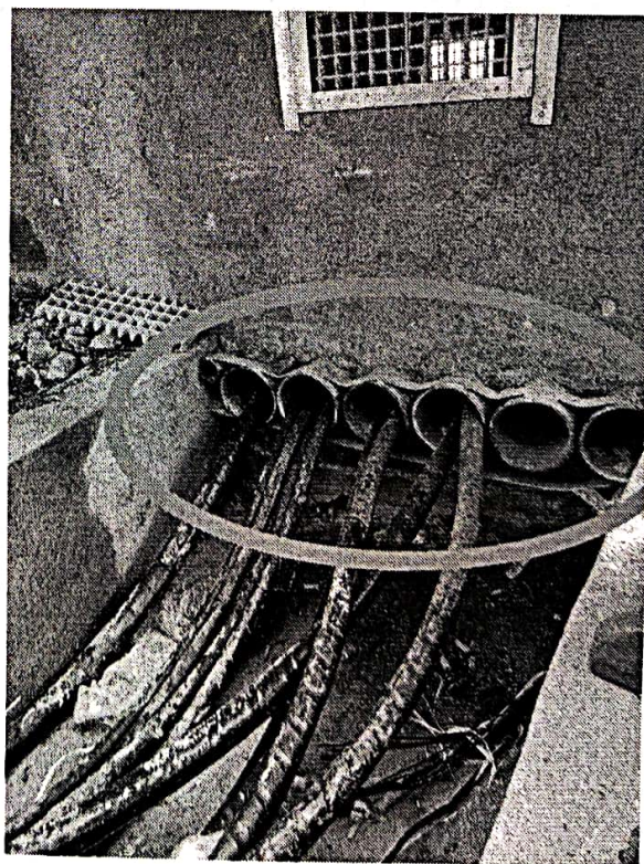
图 4：电缆穿管防火泥未封堵
