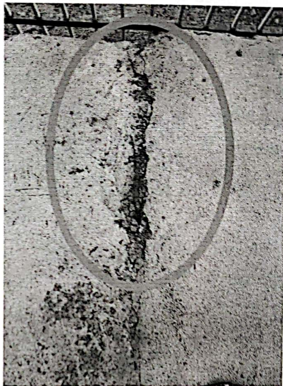
图 6：箱变基础平台施工缝未处理
