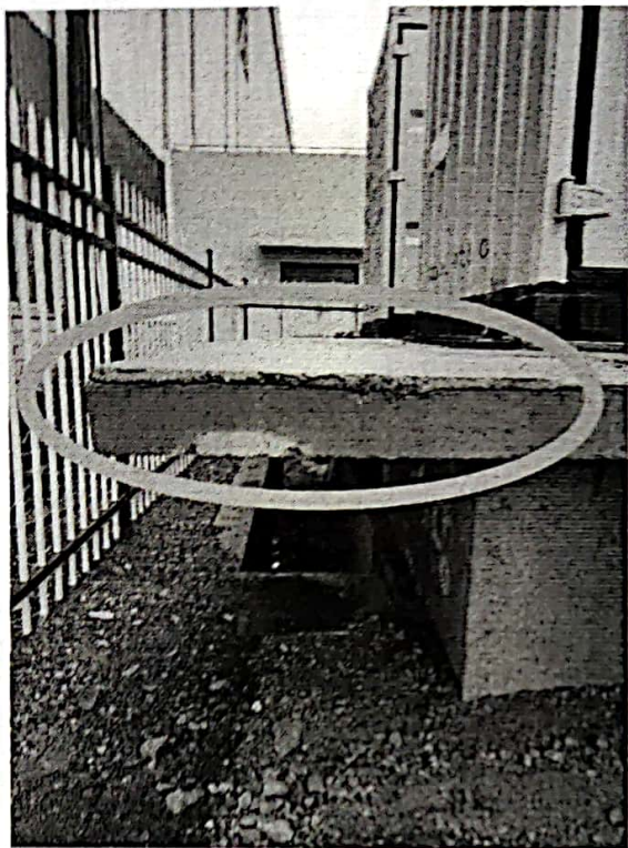
图 5：箱变基础平台抹面处理不到位
