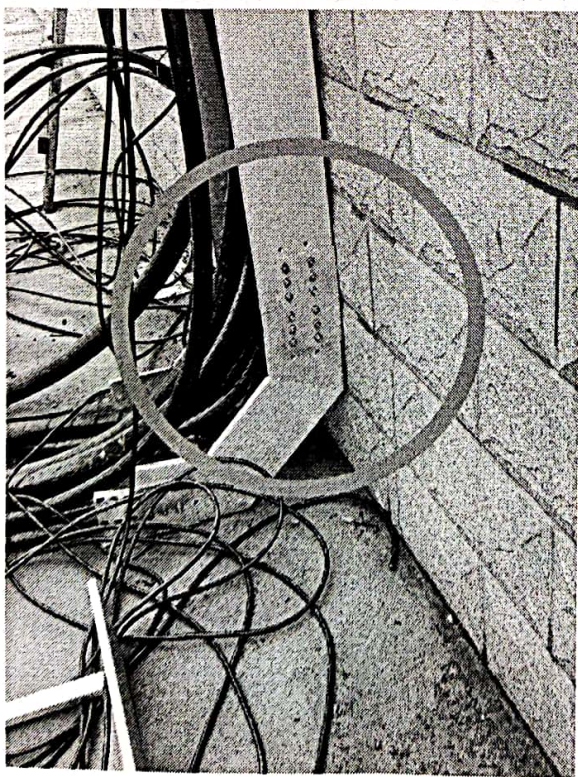
图 3：下墙桥架接地线漏接
