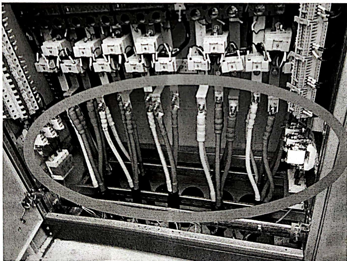
图 7：电缆未挂铭牌
