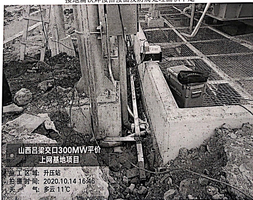
接地扁铁焊接搭接面及防腐处理面积不足
