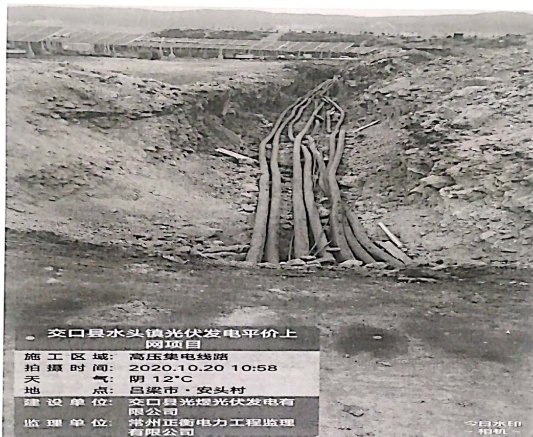
电线沟不符合规范要求
