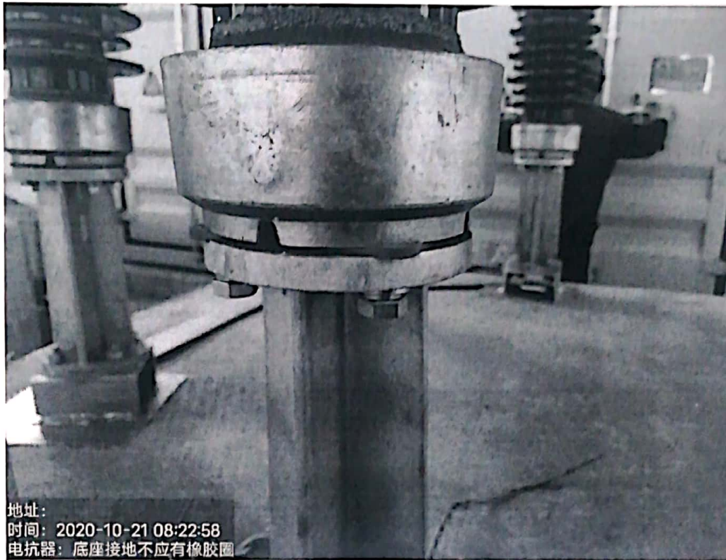
电抗器底座接地存在橡胶圈
