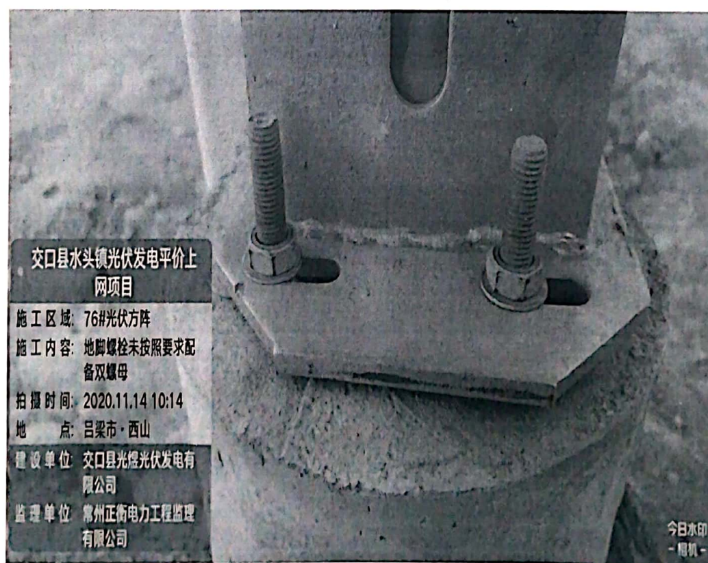
地脚螺栓未配备双螺母
