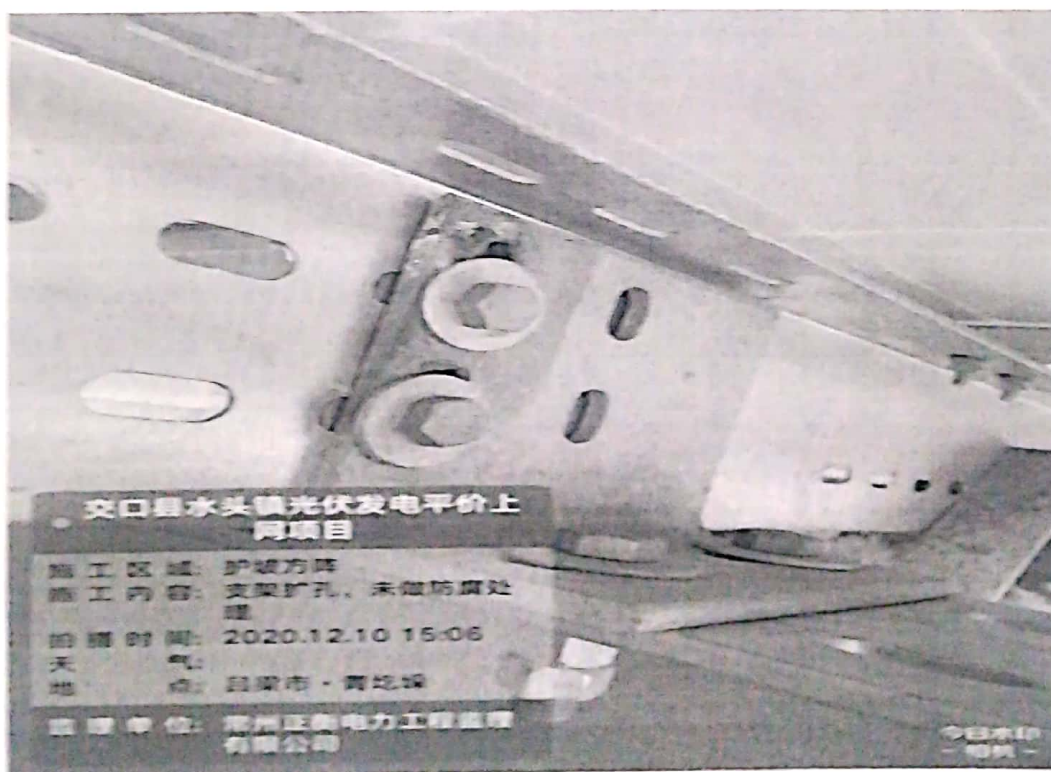
扩孔后未处理
