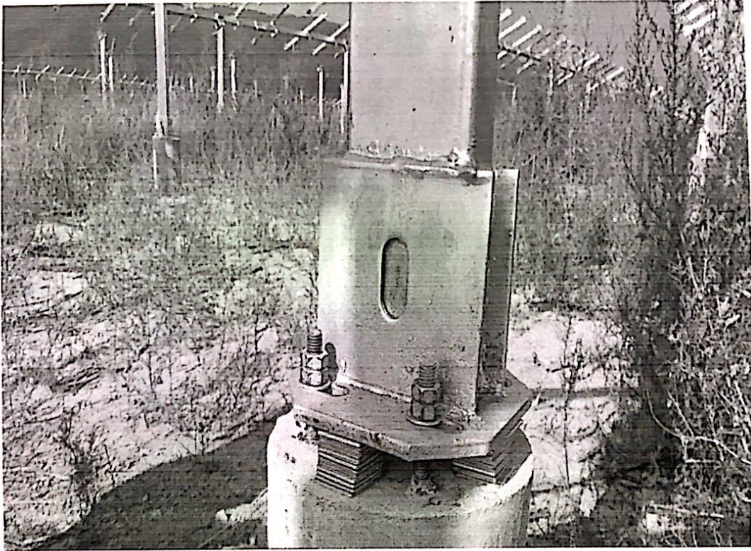
支架立柱底板未满垫、地脚螺栓未按规定使用弹垫
