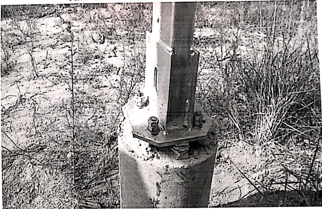
支架立柱底板未满垫、紧固螺栓外露螺丝不符合规范要求
