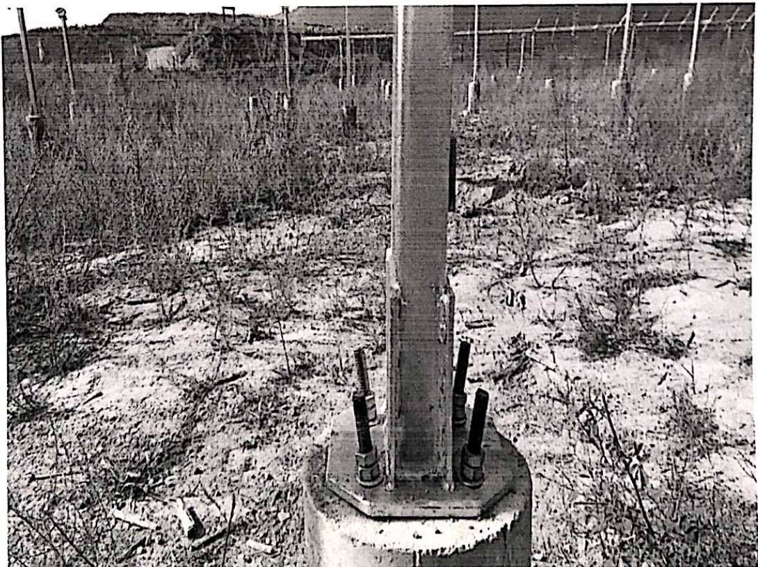
支架基础预埋件变形严重、地脚螺栓未按规定使用弹垫
