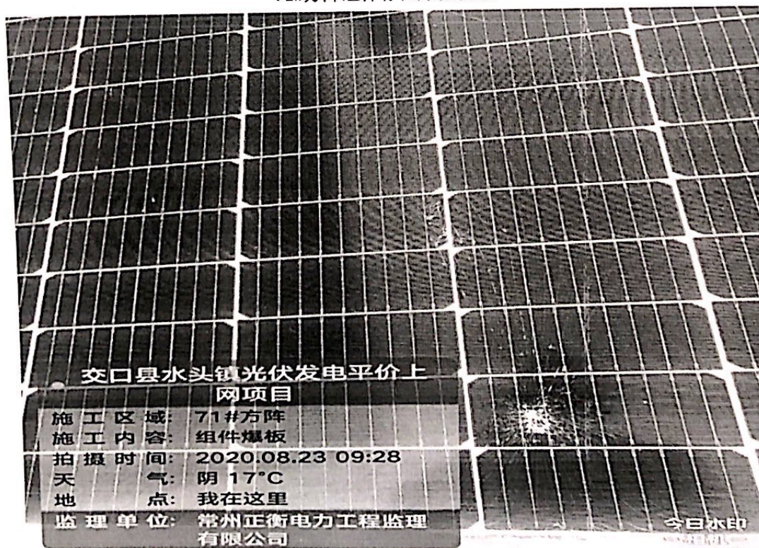
71#方阵组件存在爆板现象
